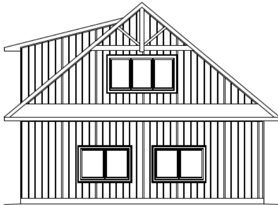
RIGHT ELEVATION
